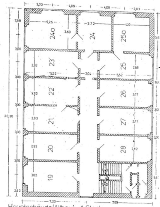
Hauptgebäude (Altbau) 1. Stock
