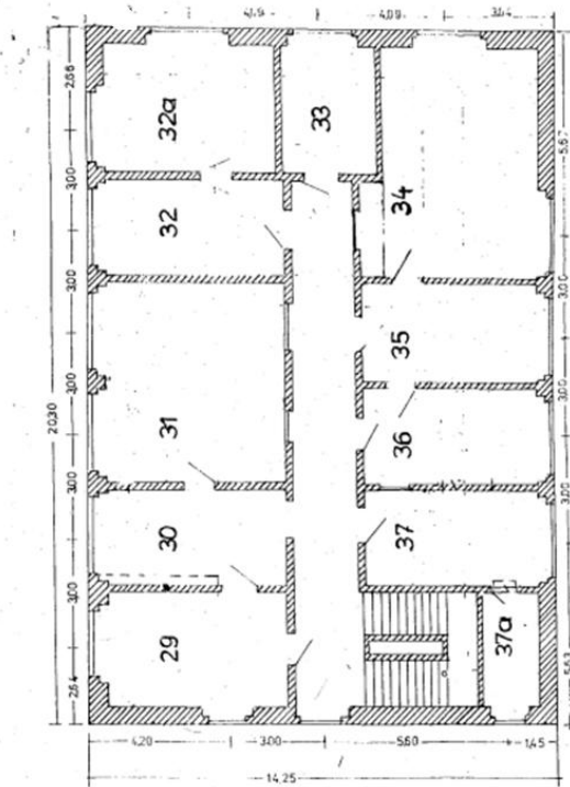
Hauptgebäude (Altbau) 2. Stock
